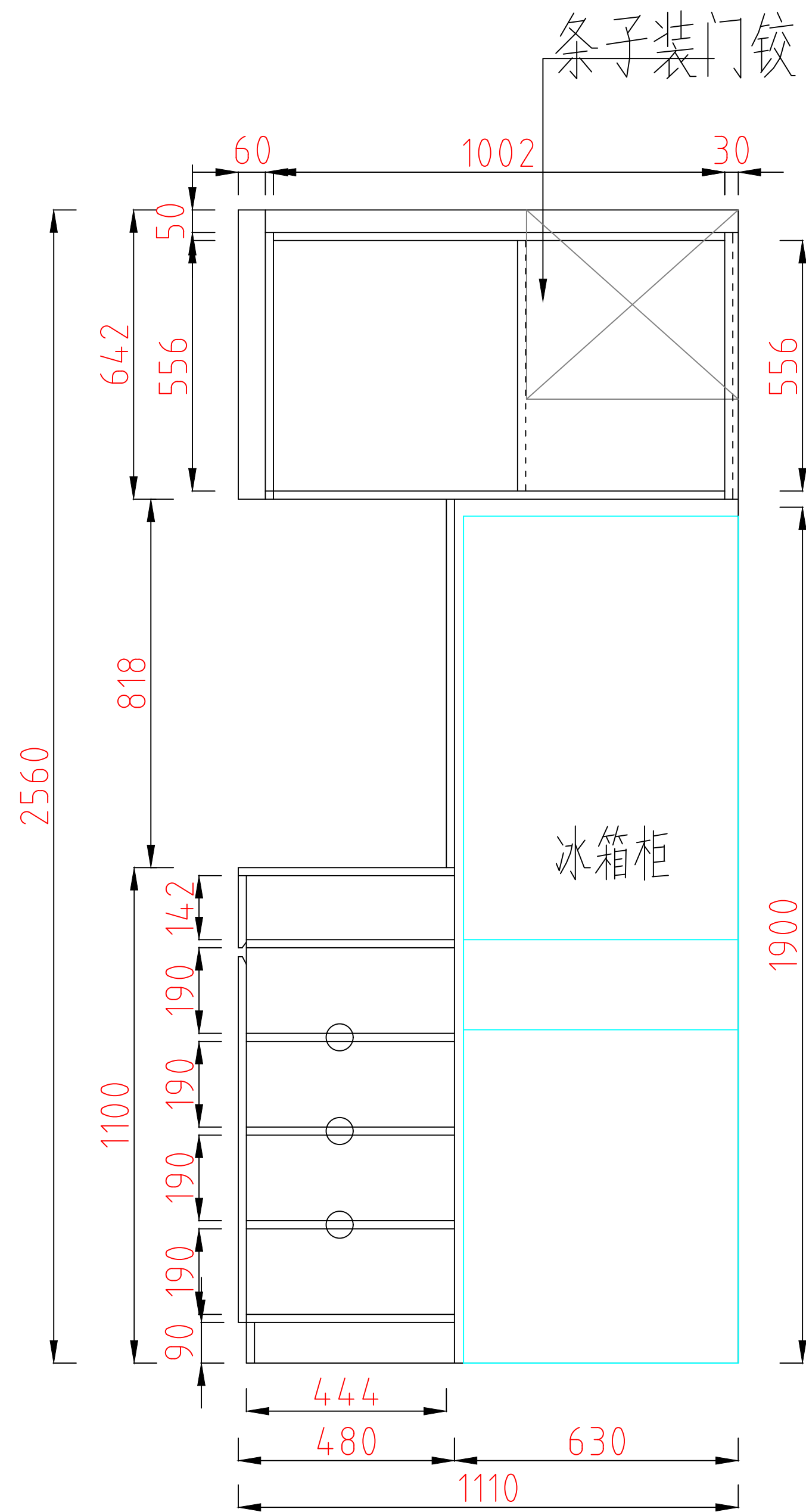
雪柜结构图
