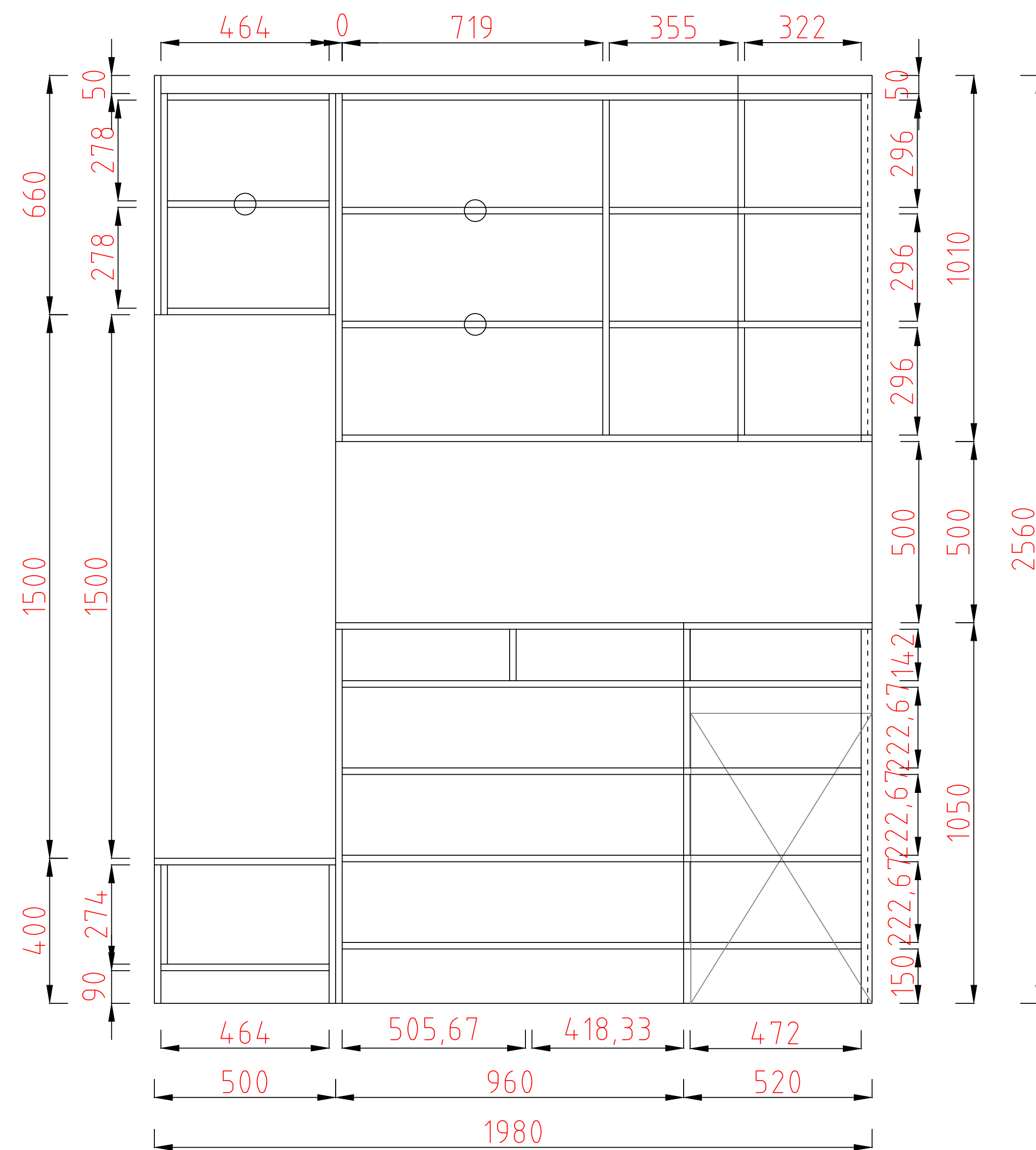
C字柜结构图
