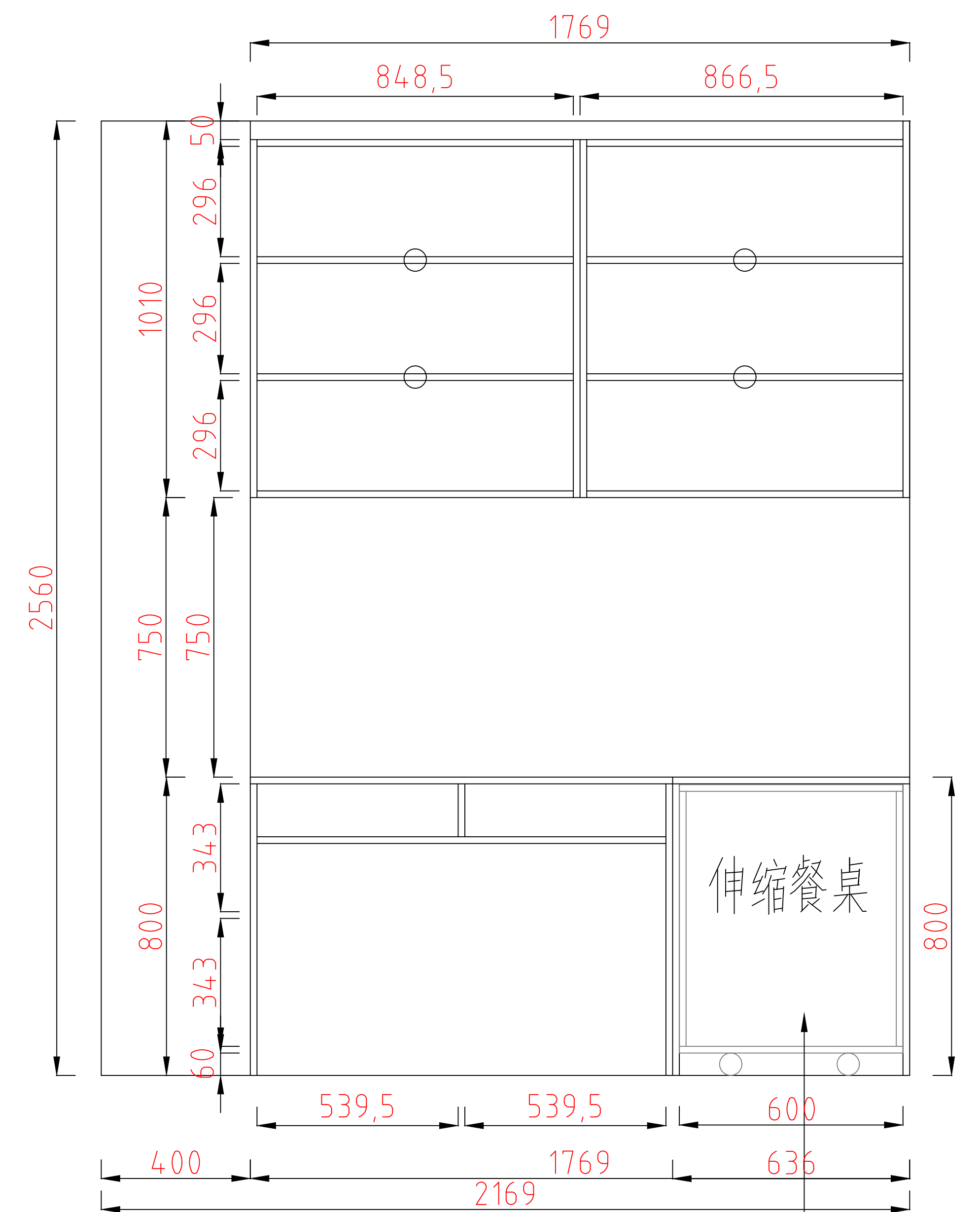
工作台加伸缩桌结构图
