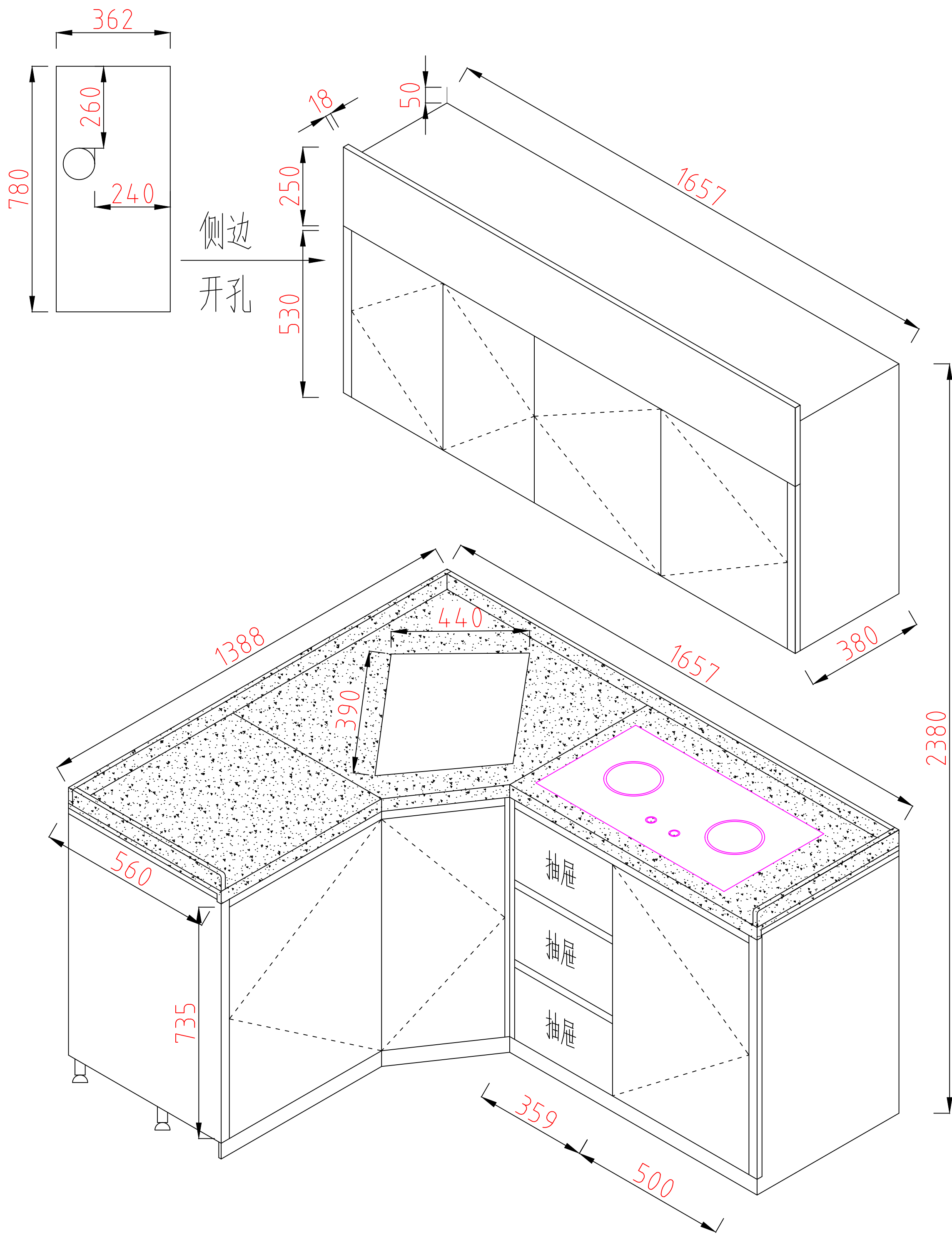
橱柜外观图
