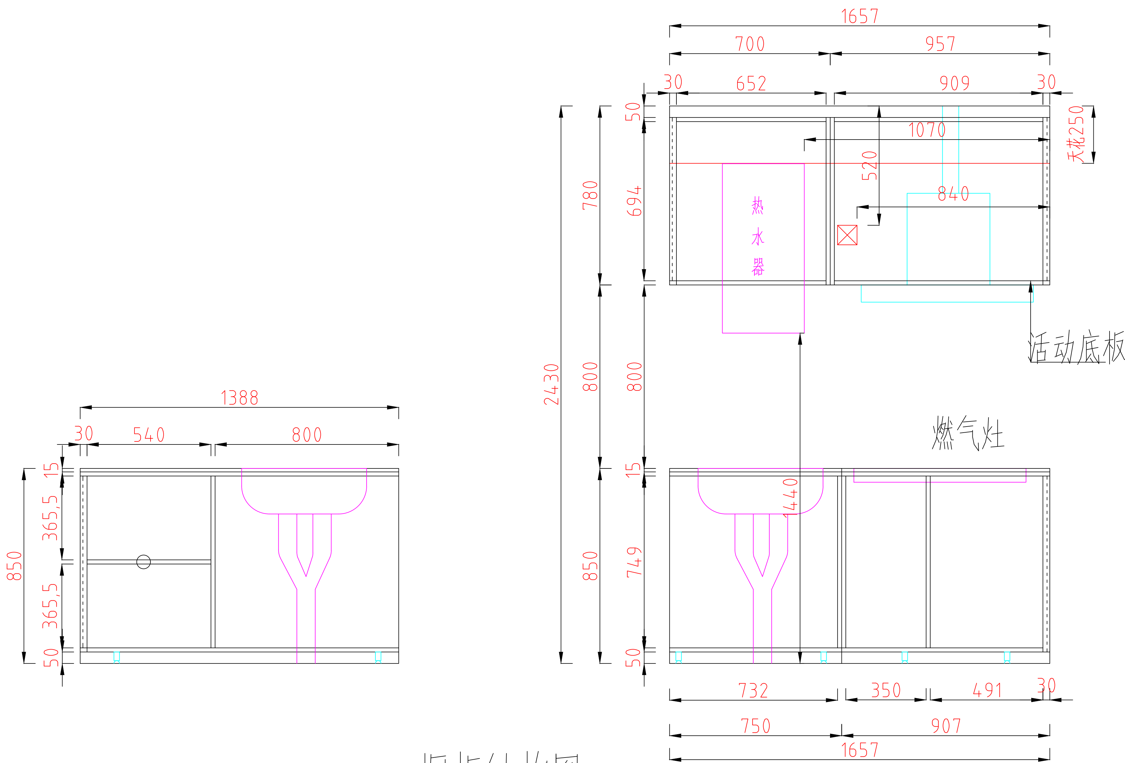
橱柜结构图
