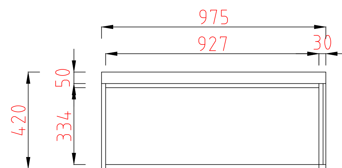
吊柜结构图
