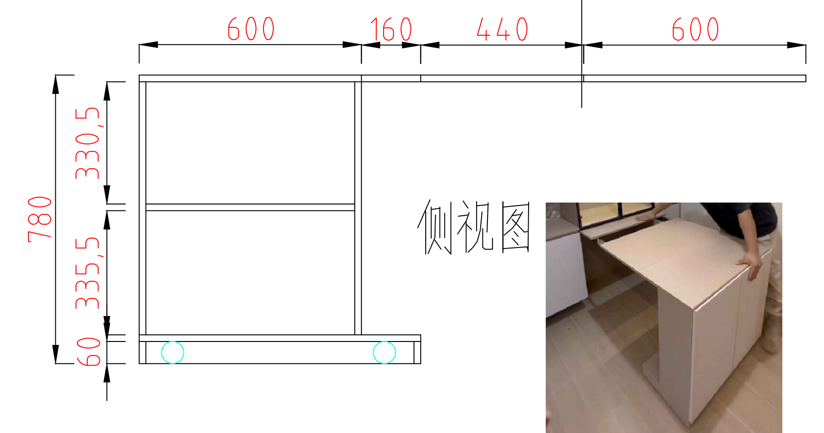
工作台加伸缩桌结构图
